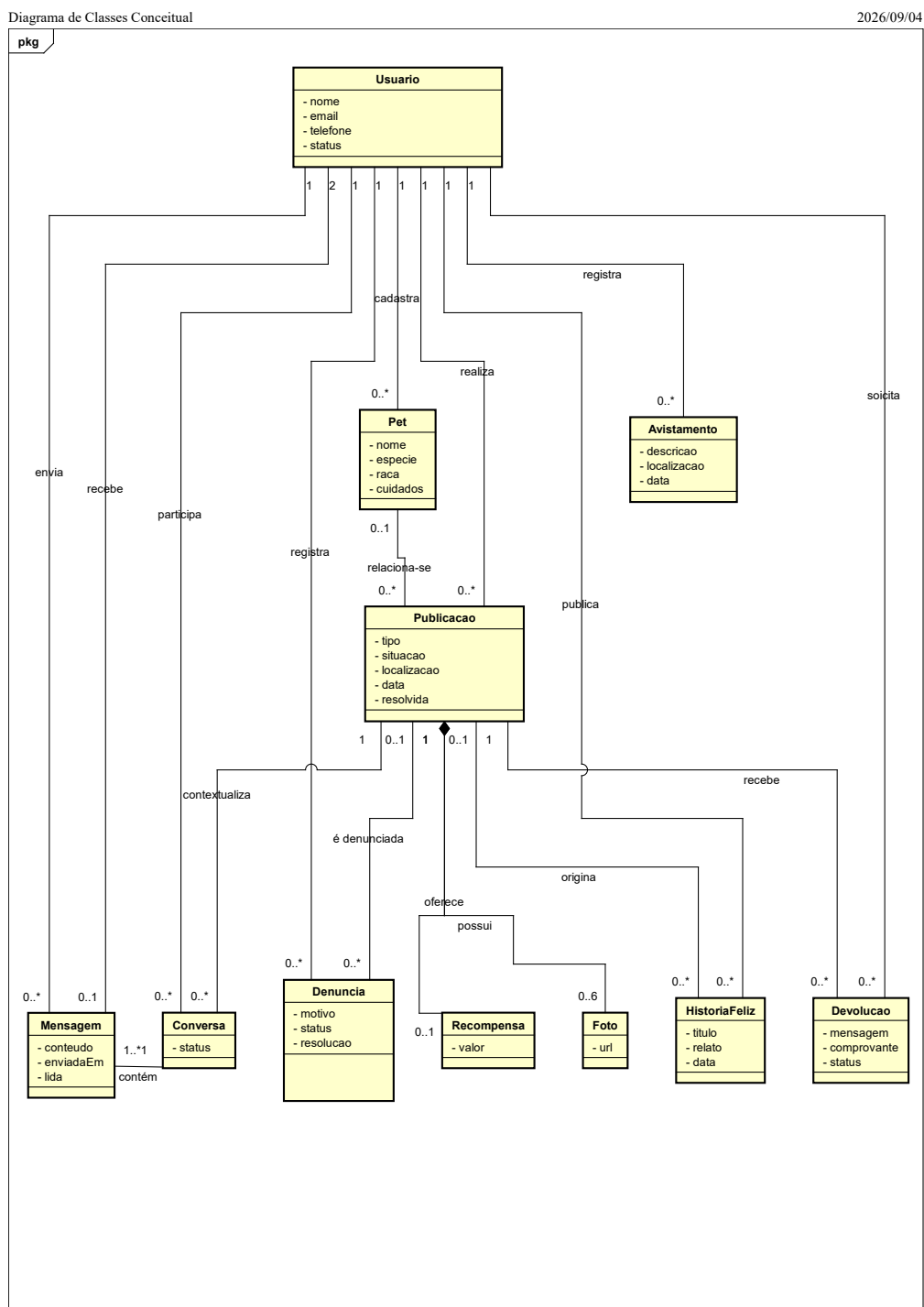
Figura 11: Diagrama de Classes Conceitual do Sistema Proposto
